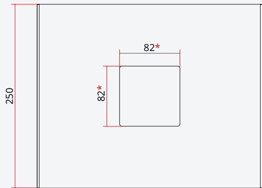
Rzut z góry Top view
