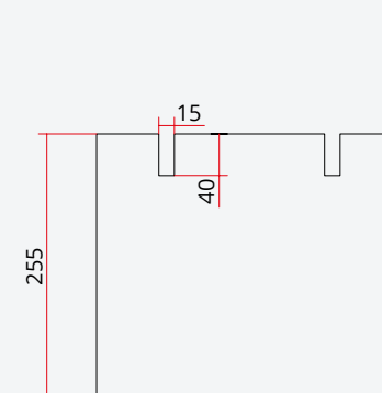
Rzut z przodu Front view
